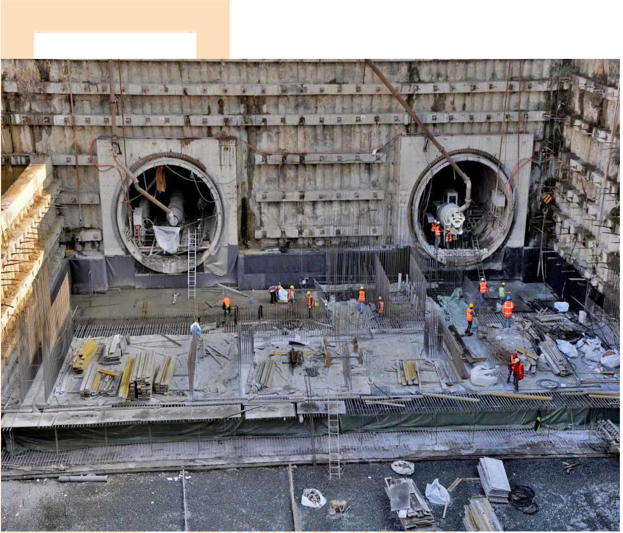
* Marmaray İnşaat Çalışmaları
